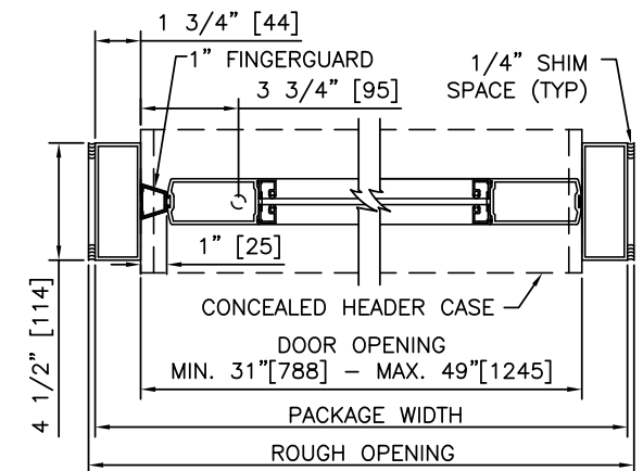
2 HORIZONTAL SECTIONS SCALE: 1 1/2" = 1'-0"
