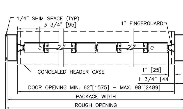
2 HORIZONTAL SECTIONS SCALE: 1 1/2" = 1'-0"
